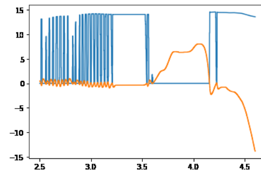
Vibrations dues à un pilotage tout ou rien (ToR)
